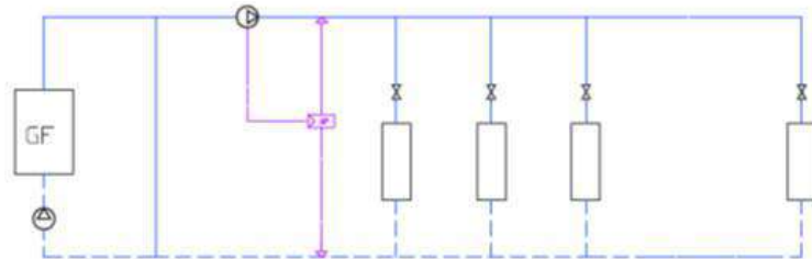
Esquema 1-a: instalación de anillo doble con refrigerador individual.
