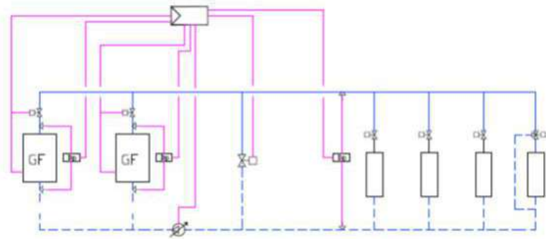
Esquema 2-b: instalación de anillo simple con caudal variable con varios refrigeradores
