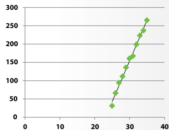
VARIACIÓN DE CAUDAL/POTENCIA BATERÍA ON-OFF (FAN COIL)
