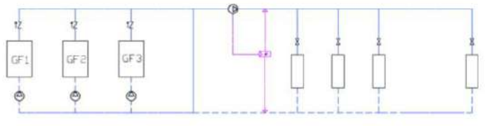
Esquema 1-b: instalación de anillo doble con varios refrigeradores en paralelo.
