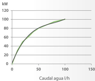
VARIACIÓN DEL CAUDAL/POTENCIA BATERÍA MODULADORA (UTA)
