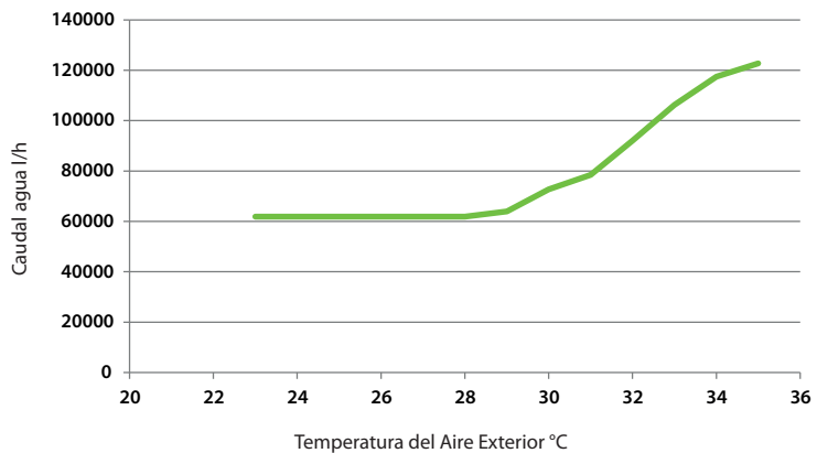
Caudal de agua medio de la bomba VPF en función de la temperatura externa
