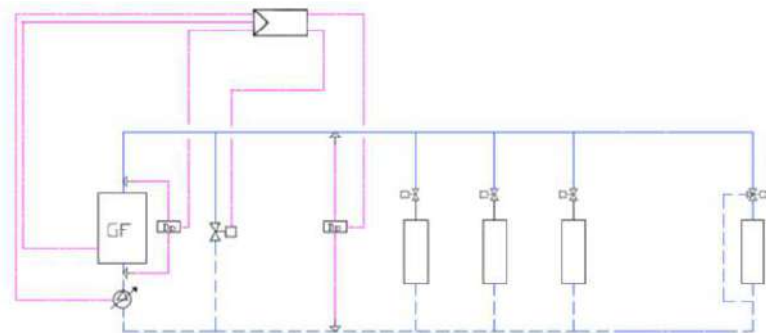
Esquema 2-a: instalación de anillo simple con caudal variable con un solo refrigerador
